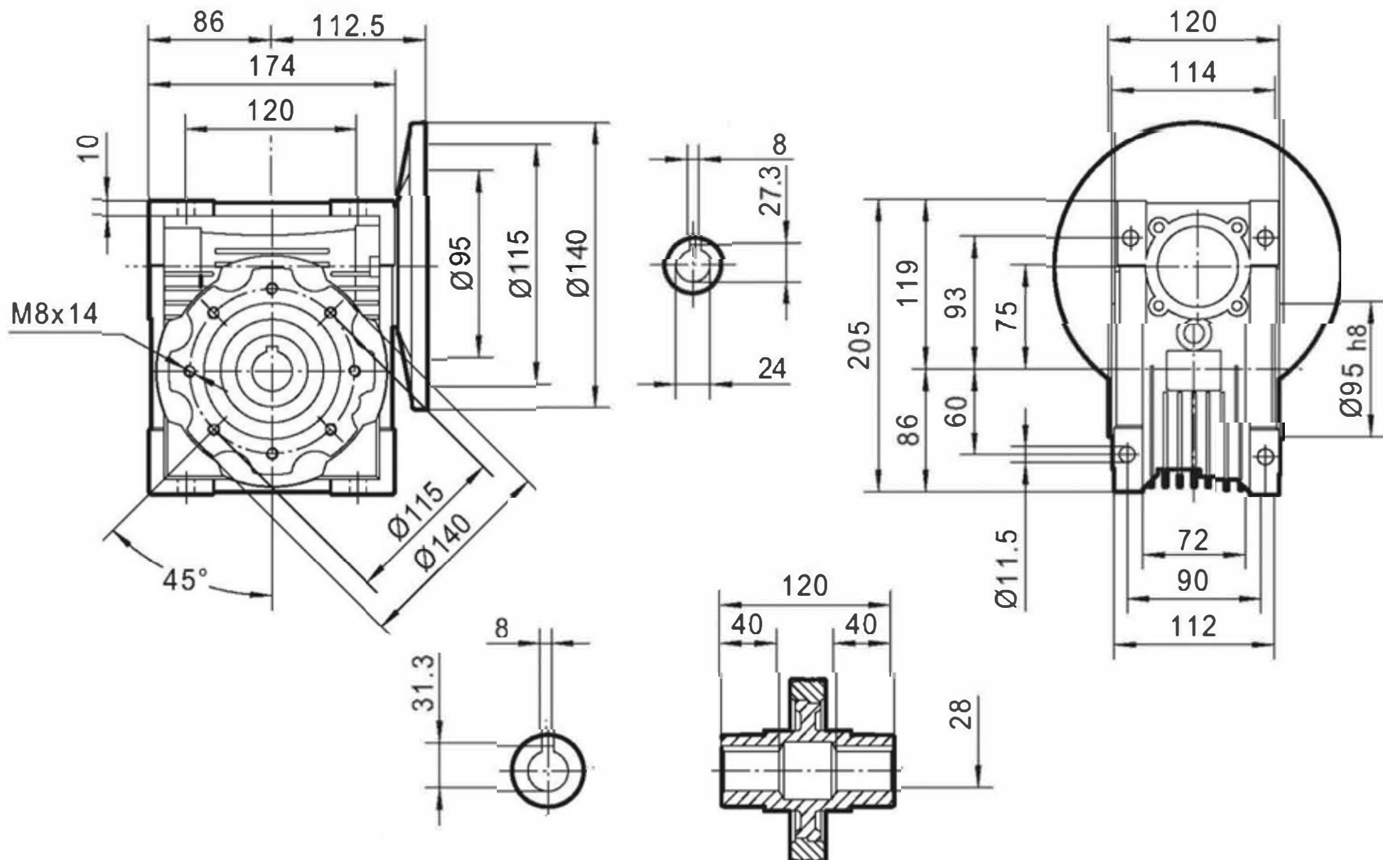
NMRV 075 90B14
