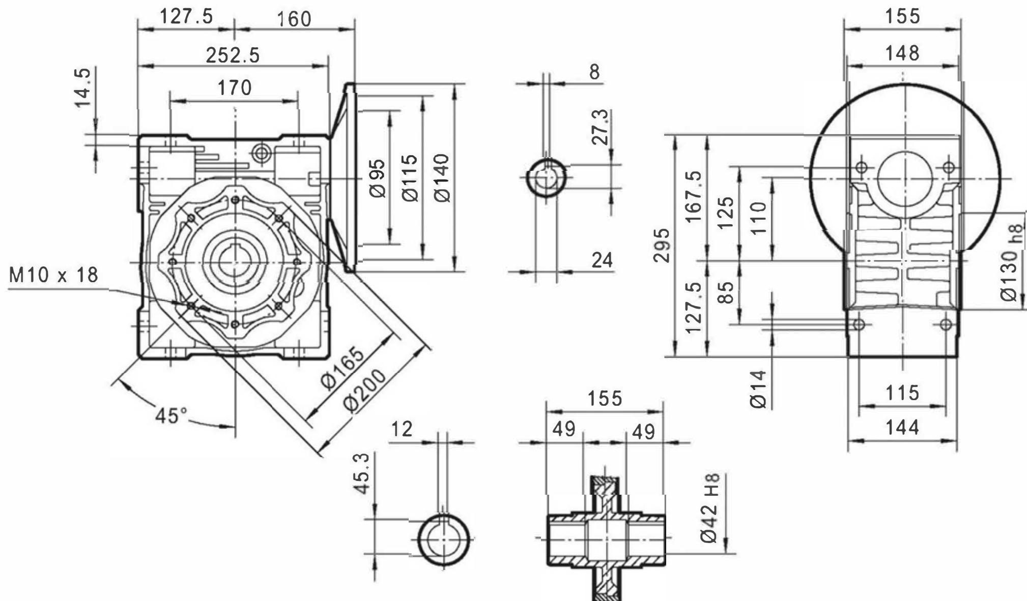
NMRV 110 90B14
