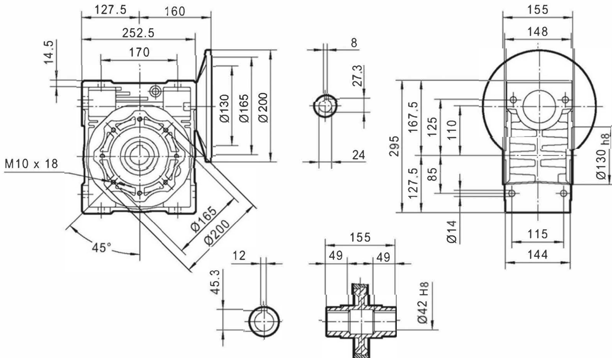
NMRV 110 90B5
